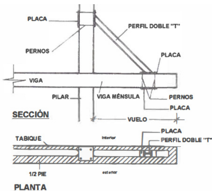
Fig 2.- Reparación oculta en el cerramiento.
